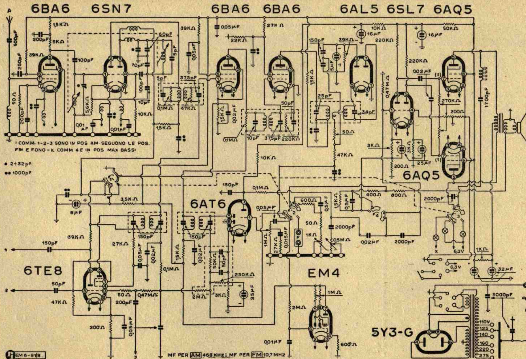
Lo schema elettrico del Mod. 4110 AM-FM N.B. - Vedere a tergo schema elettrico del gruppo AF
